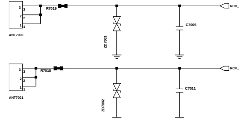
RCV CONTACT
